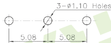
P.C.B layout
