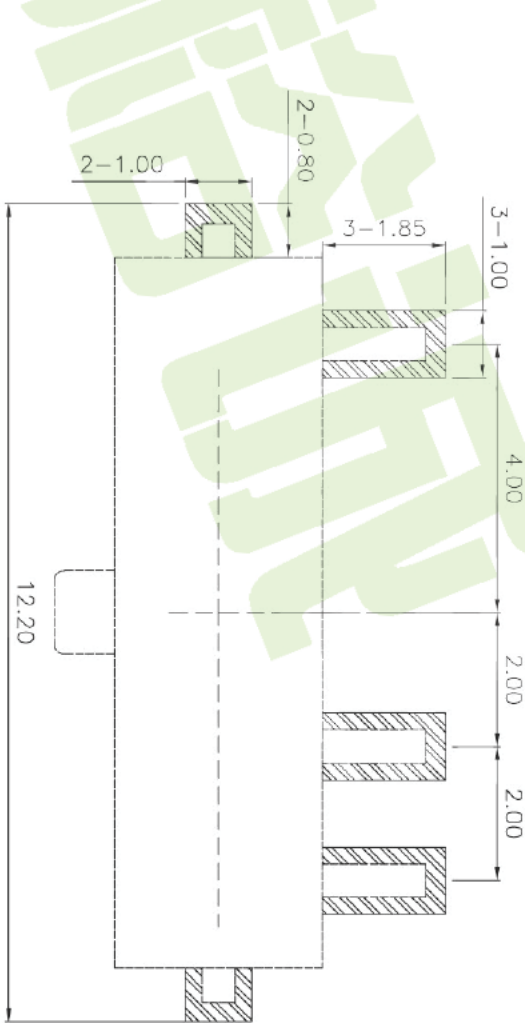
P.C.B layout
